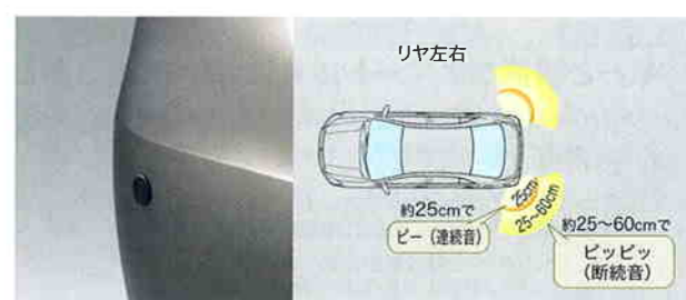
032 コーナーセンサー(リヤ左右)
